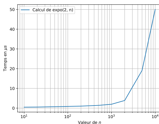
FIGURE 5.8 – Graphique semilog pour l'exponentiation rapide d'un entier.
