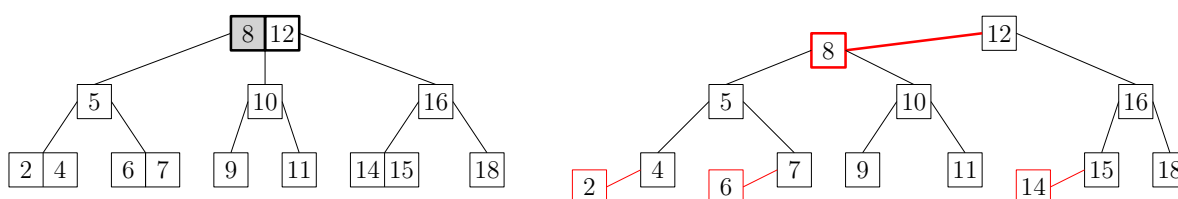
FIGURE 11.35 – Le problème se transmet au niveau supérieur, et disparaît.
