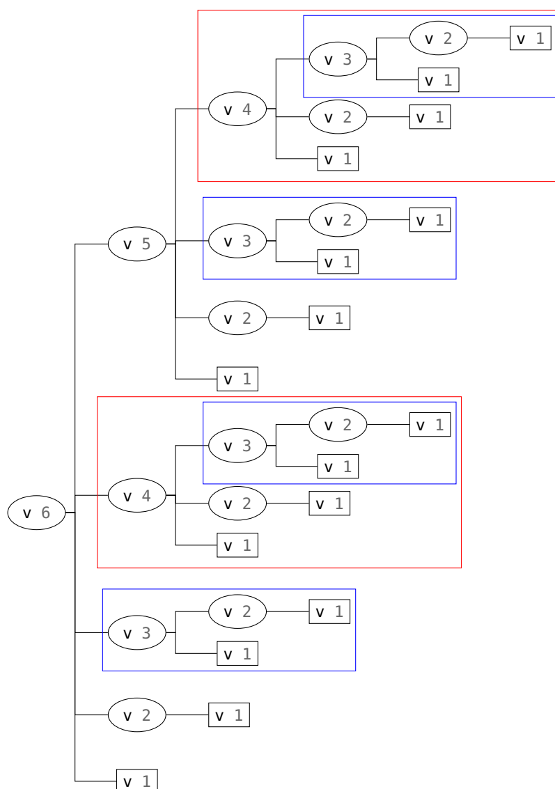
FIGURE 13.8 – Découpage optimal pour n = 6 , récursif naïf. Les sous-arbres encadrés d'une même couleur sont identiques.
