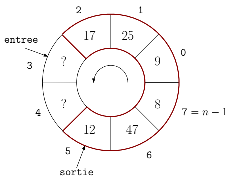
FIGURE 7.11 – La file f = (17, 25, 9, 8, 47, 12) dans un tableau de capacité 8.
