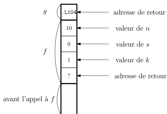
FIGURE 8.2 – État de la pile d'appels lors du premier passage ligne 8 dans le calcul de f 10 .
