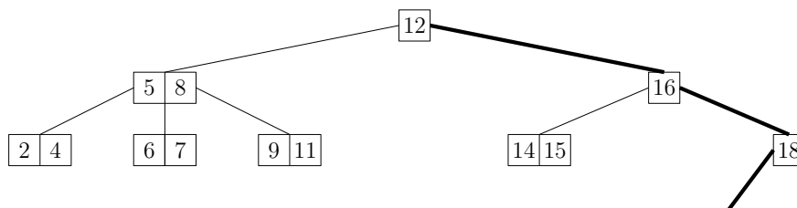
FIGURE 11.14 – Insertion de 17, recherche de l'emplacement.
