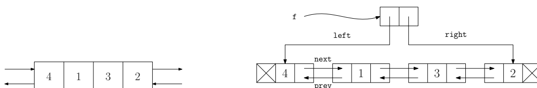
FIGURE 7.17 – La deque (4, 1, 3, 2) et sa réalisation sous forme de liste doublement chaînée.
