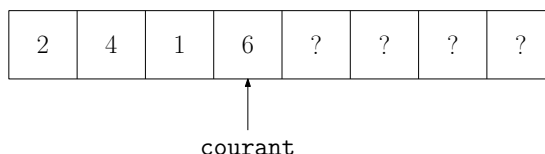
FIGURE 7.5 – Une pile de capacité 8 contenant quatre éléments. courant vaut 3, donc le sommet de la pile est donnees.(3) = 6 .
