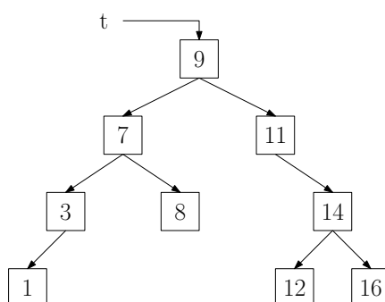
FIGURE 11.6 – Un ABR t (en C ou en OCaml).
