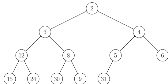
FIGURE 12.10 – Après insertion de 5.
