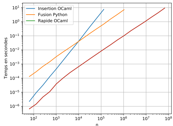
FIGURE 5.7 – Comparaison de temps de calcul.
