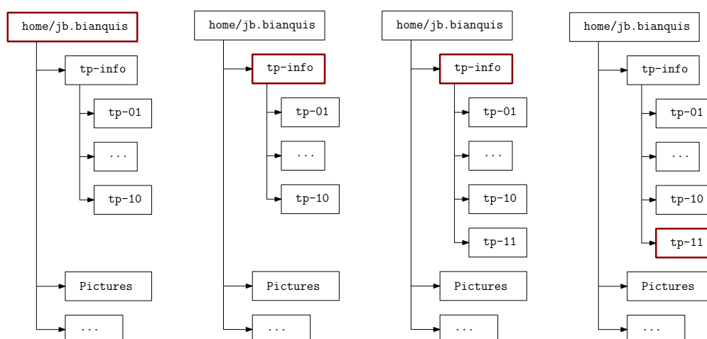
FIGURE XI.1 – Évolution de l'arborescence lors de l'exécution des commandes ci-dessus. Le répertoire en gras est le répertoire courant.
