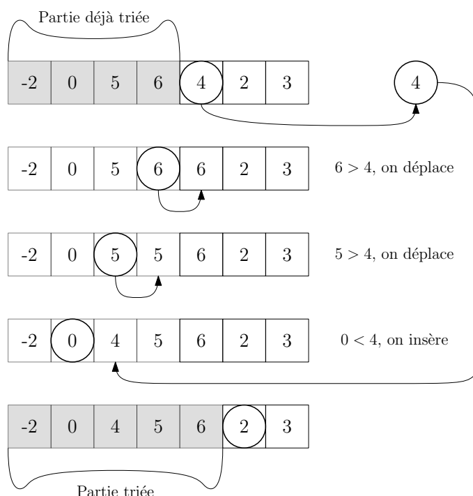
FIGURE IV.2 – Insertion avec deux fois moins d'écritures.
