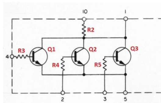
FIGURE 16.2 – Schéma électronique équivalent. La patte 5 est V_0 , 10 est V_+ , 1 est le NOR de 2, 3 et 4. Le schéma est le même pour les pattes 6 à 9.
