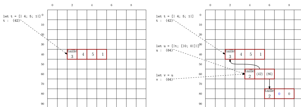
FIGURE 6.5 – Représentation mémoire des array en OCaml.
