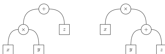
FIGURE 10.11 – Les deux arbres ci-dessus admettent exactement le même parcours en profondeur infixe : x \times y + z . En revanche, leurs parcours préfixes (ou suffixes) sont distincts.
