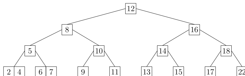
FIGURE 11.24 – Insertion de 22, état final après scission de la racine.
