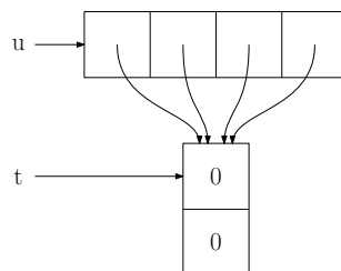
FIGURE 3.4 – Schéma-mémoire après let u = Array.create 4 t .
