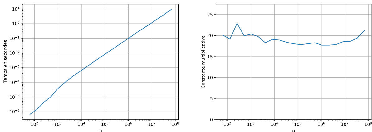
FIGURE 5.2 – Tri rapide en OCaml (raisonnablement optimisé).
