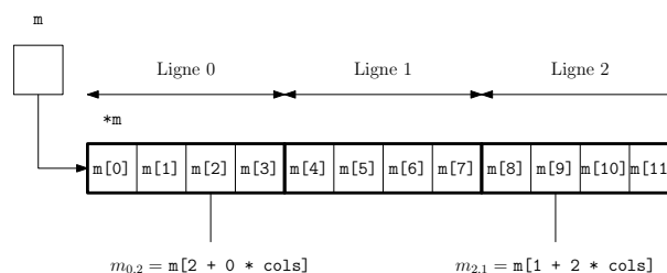
FIGURE 8.9 – Tableau bidimensionnel à plat, format row major .
