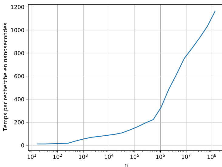
FIGURE 5.5 – Si le temps par recherche était proportionnel à \log n , on obtiendrait une droite.
