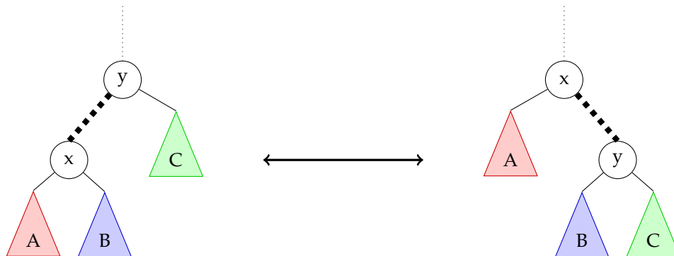
FIGURE 11.36 – Rotation autour de l'arête xy.
