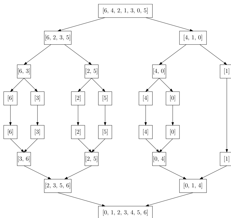
FIGURE IV.4 – Détail du tri fusion
