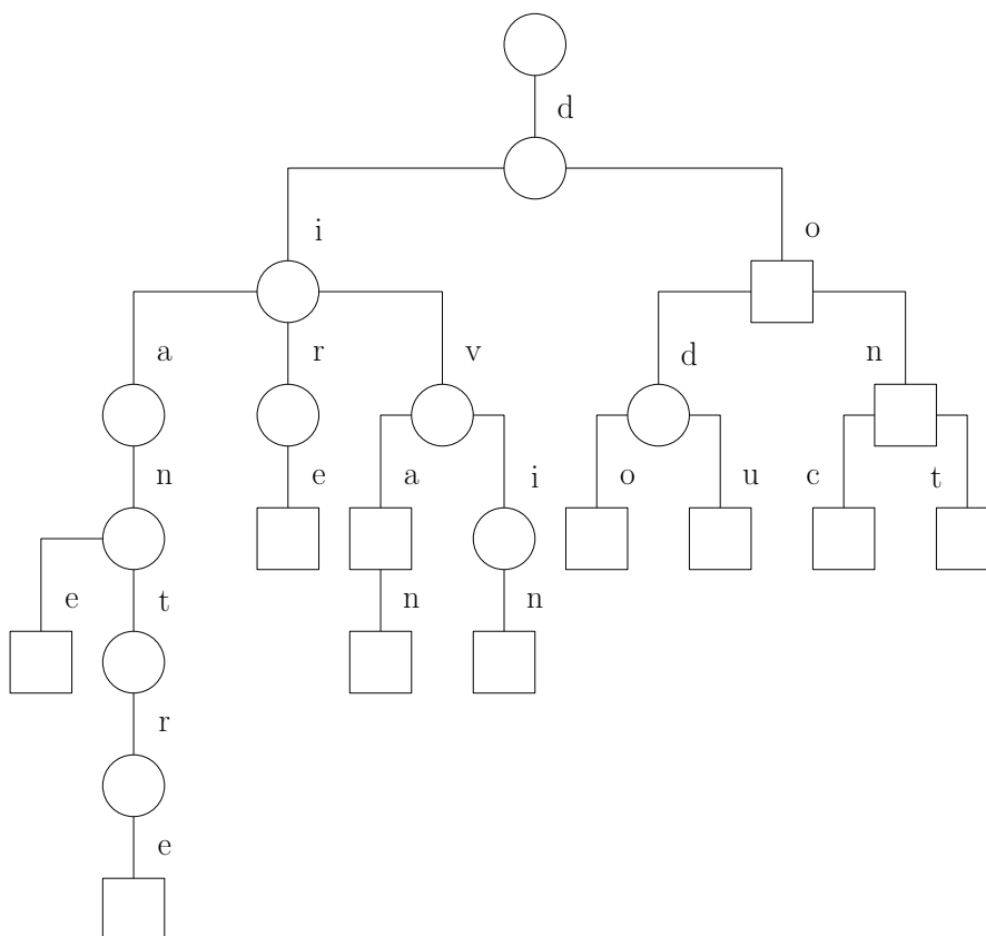
FIGURE 10.3 – Un trie pour l'ensemble \{\text{diane, diantre, dire, diva, divan, divin, do, dodo, dodu, don, donc, dont}\} .
