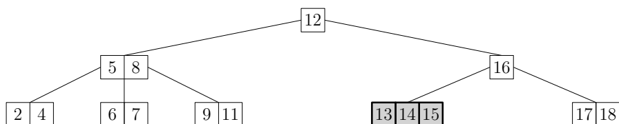
FIGURE 11.16 – Insertion de 13, étape intermédiaire.
