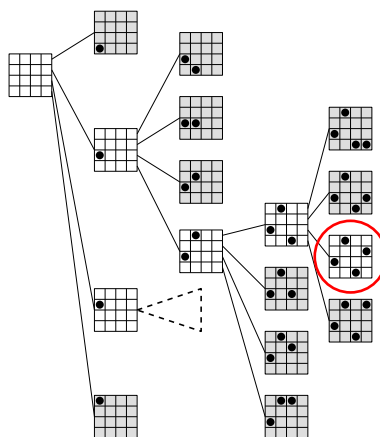
FIGURE 17.5 – Arbre obtenu avec une règle de rejet parfaite.
