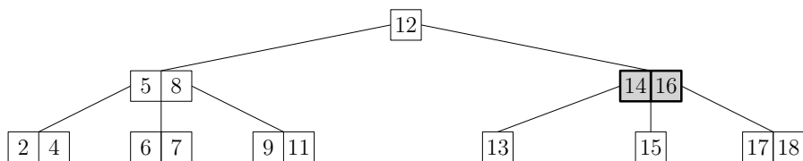
FIGURE 11.17 – Insertion de 13, suppression du nœud quaternaire.
