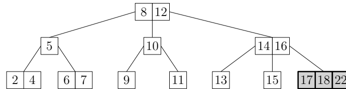
FIGURE 11.21 – Insertion de 22, première étape.
