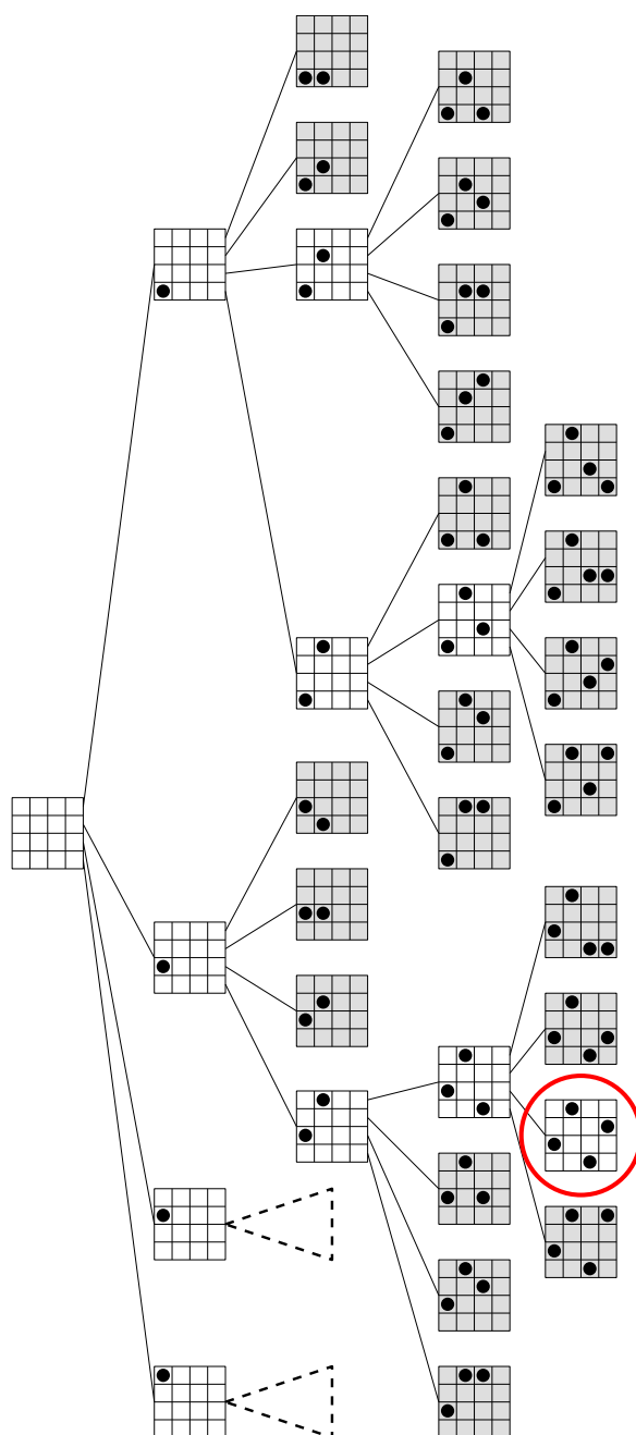
FIGURE 17.2 – Arbre exploré pour le problème des 4 dames. Seule la moitié a été représentée, l'autre est symétrique; la solution est entourée (il y en a une autre dans la partie symétrique), les candidats (complets ou non) rejetés sont grisés.
