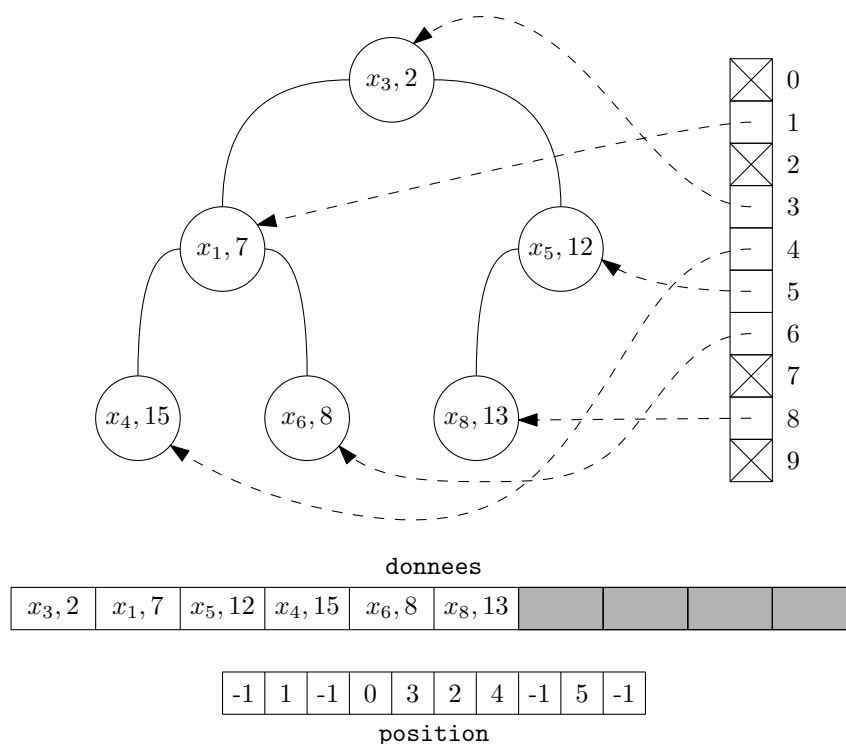
FIGURE 15.9 – Tas binaire avec tableau indiquant la position des clés.
