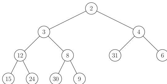
FIGURE 12.9 – Après insertion de 2.
