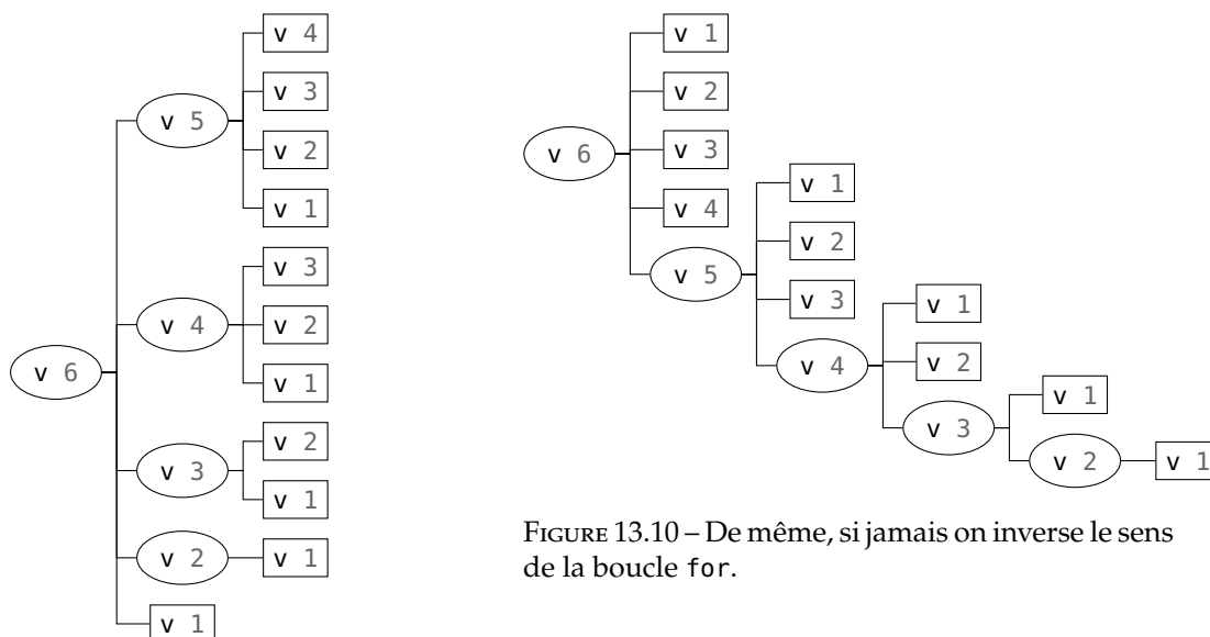
FIGURE 13.9 – Découpage de toblerone pour n = 6 , récursif mémorisé.
