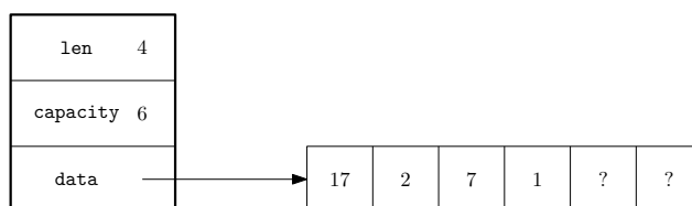
FIGURE XVI.2 – Un int_dynarray_t de capacité 6 contenant 4 éléments.
