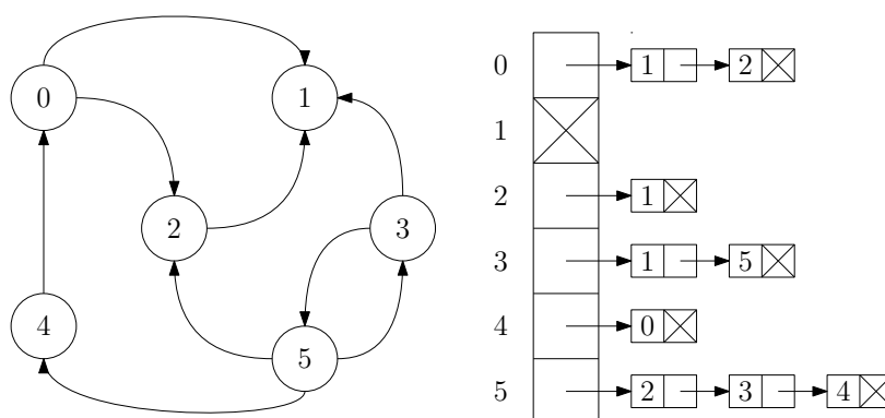
FIGURE 15.1 – Un graphe orienté et le tableau de listes d'adjacence correspondant.
