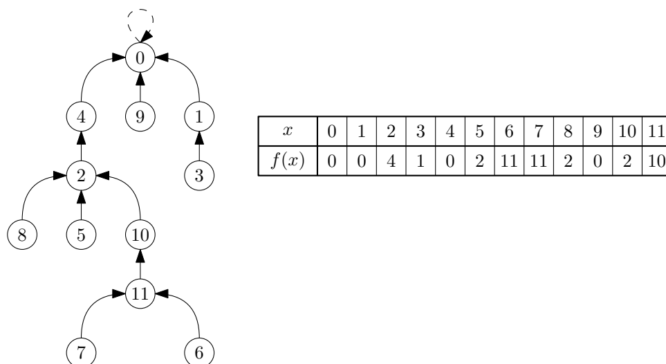
FIGURE 14.43 – Une application nilpotente et l'arbre enraciné correspondant.
