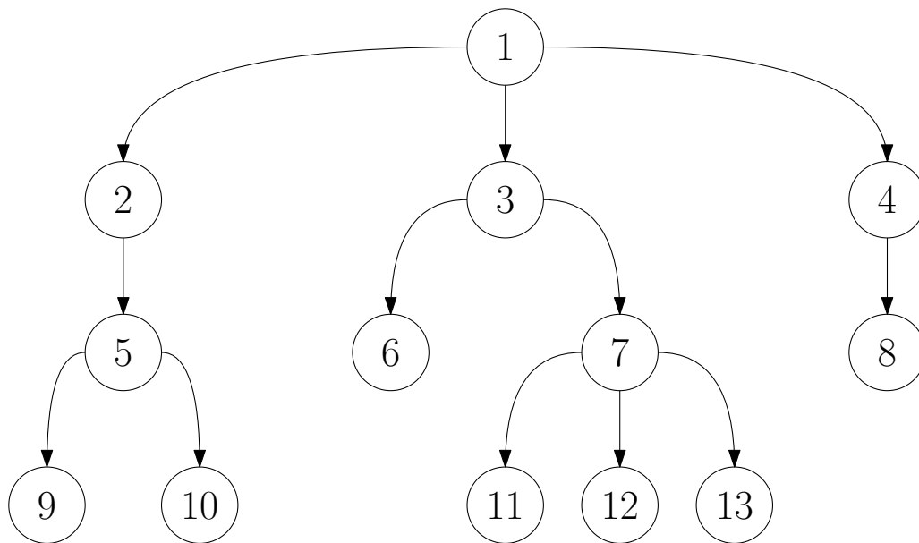
FIGURE 10.1 – L'arbre T
