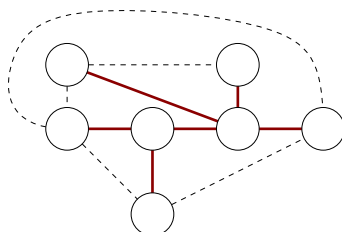
FIGURE 14.18 – Un graphe et l'un de ses arbres couvrants (arêtes en gras).
