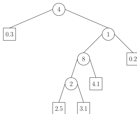
FIGURE XXI.1 – L'arbre exemple2.
