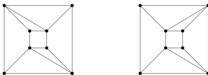
FIGURE 14.14 – Les graphes H_1 et H_2 .
