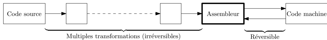
FIGURE 8.3 – Étapes de la compilation d'un programme OCaml.
