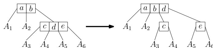
FIGURE 11.43 – Fils droit d'un nœud ternaire.
