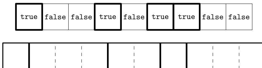
FIGURE 13.6 – La découpe 1, 3, 2, 1, 3 et le tableau de booléens correspondant.
