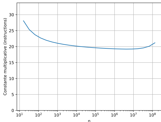
FIGURE 5.3 – Le nombre d'instructions par recherche vaut environ 20 \log n .
