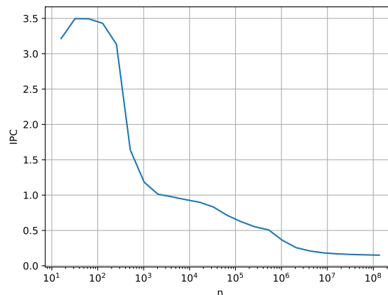
FIGURE 5.4 – Le nombre d'instructions par cycle décroît fortement avec n .
