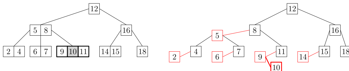
FIGURE 11.33 – Création d'une feuille rouge.
