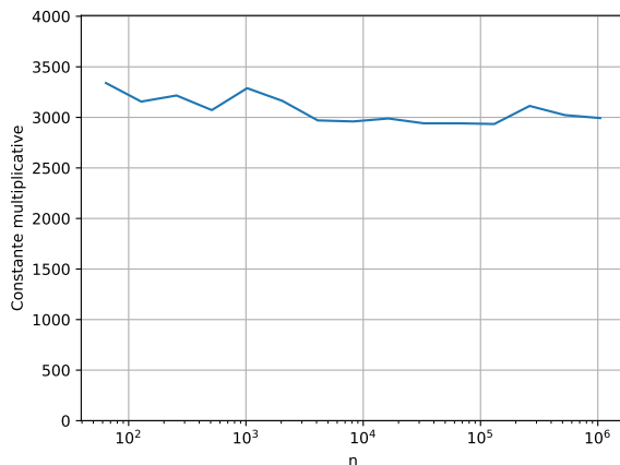
FIGURE 5.6 – Le nombre d’instructions exécutées par cette variante du tri fusion en Python est de l’ordre de 3000n \log n .
