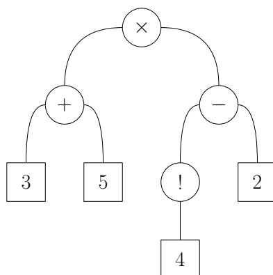
FIGURE 10.2 – L'arbre de l'expression (3 + 5) \times (4! - 2) .
