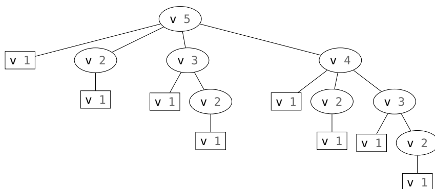
FIGURE 13.7 – Découpage de toblerone pour n = 5 , récursif naïf
