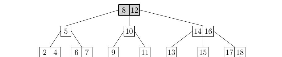
FIGURE 11.20 – Insertion de 10, état final.
