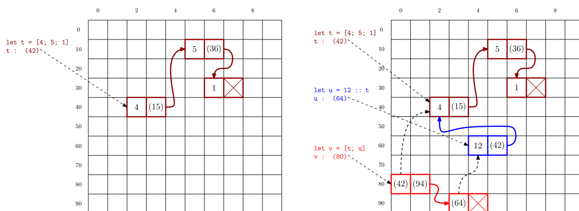
FIGURE 6.7 – Représentation mémoire des list en OCaml.
