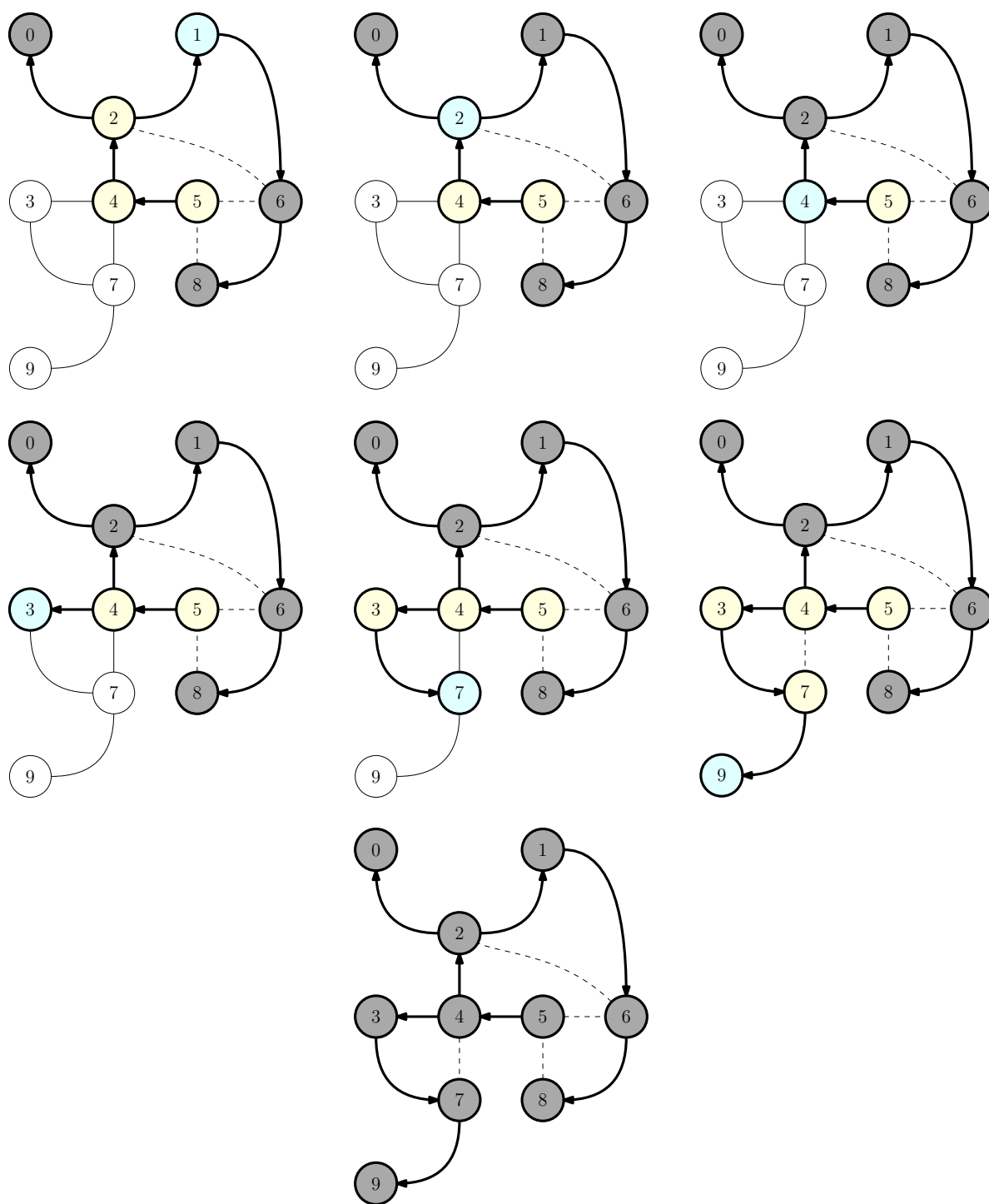
FIGURE 15.2 – Parcours en profondeur d'un graphe connexe non orienté.
