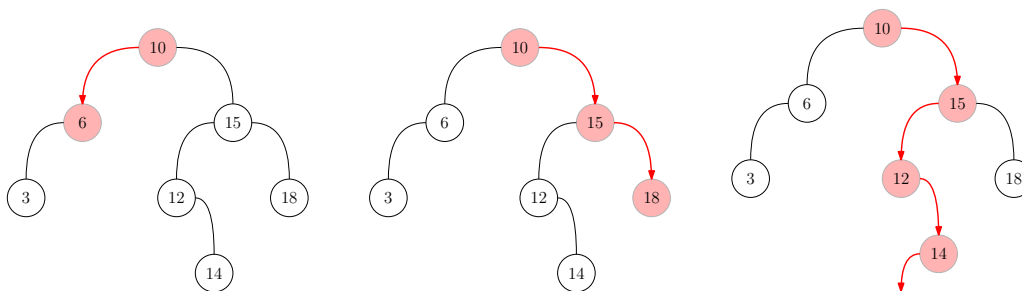
FIGURE 11.5 – Recherche de 6, de 18 et de 13 dans un ABR
