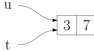
FIGURE 3.3 – Schéma-mémoire après let u = t .
