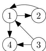
FIGURE 14.9 – Un exemple de matrice d'adjacence pour un graphe orienté.
