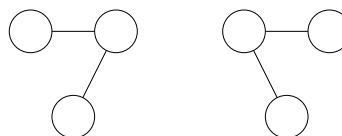
FIGURE 14.27 – Deux graphes non étiquetés identiques.
