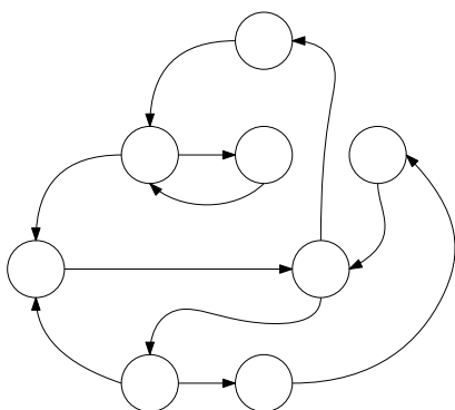
FIGURE 14.20 – Un graphe fortement connexe.
