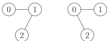
FIGURE 14.26 – Deux graphes étiquetés distincts.
