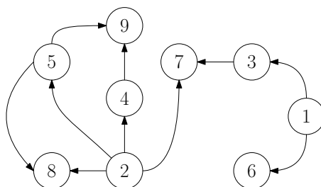
FIGURE 14.22 – Un exemple de DAG.
