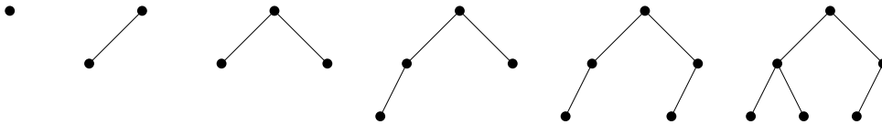
FIGURE XXX.1 – Arbres de Braun à 1, 2, ..., 6 nœuds.
